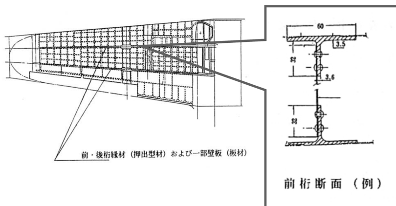
図4 零戦主翼の図版と主桁前桁の断面図 19)
