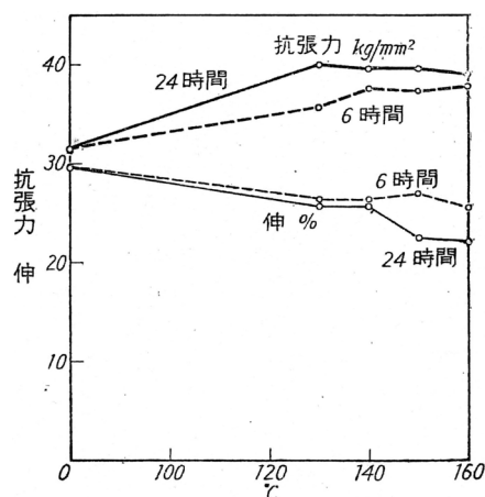
図6 25Sの高温時効特性 34)
