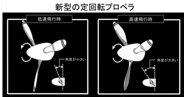
図5 定回転プロペラのピッチ角度 14)
